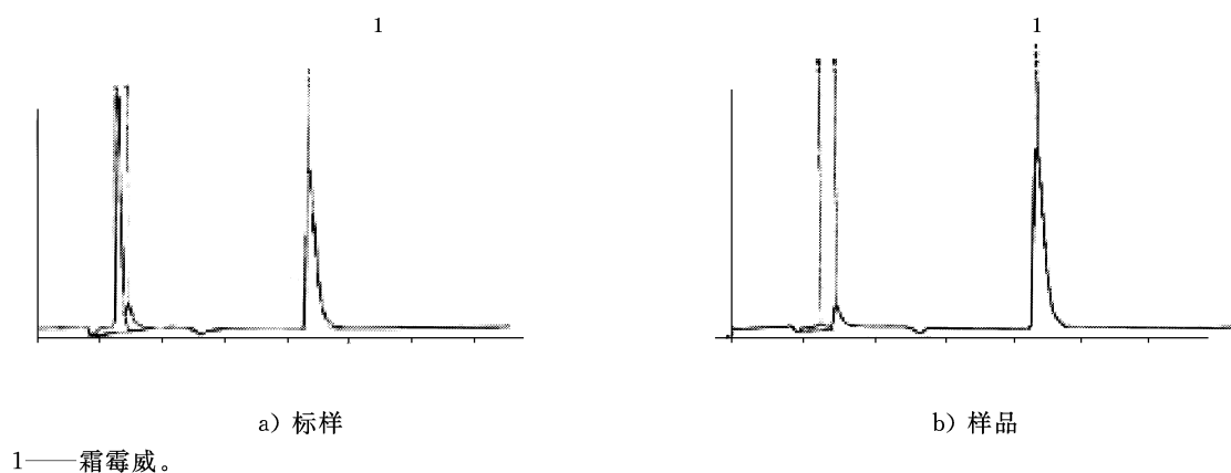
图 A.1 霜霉威原药的液相色谱图
